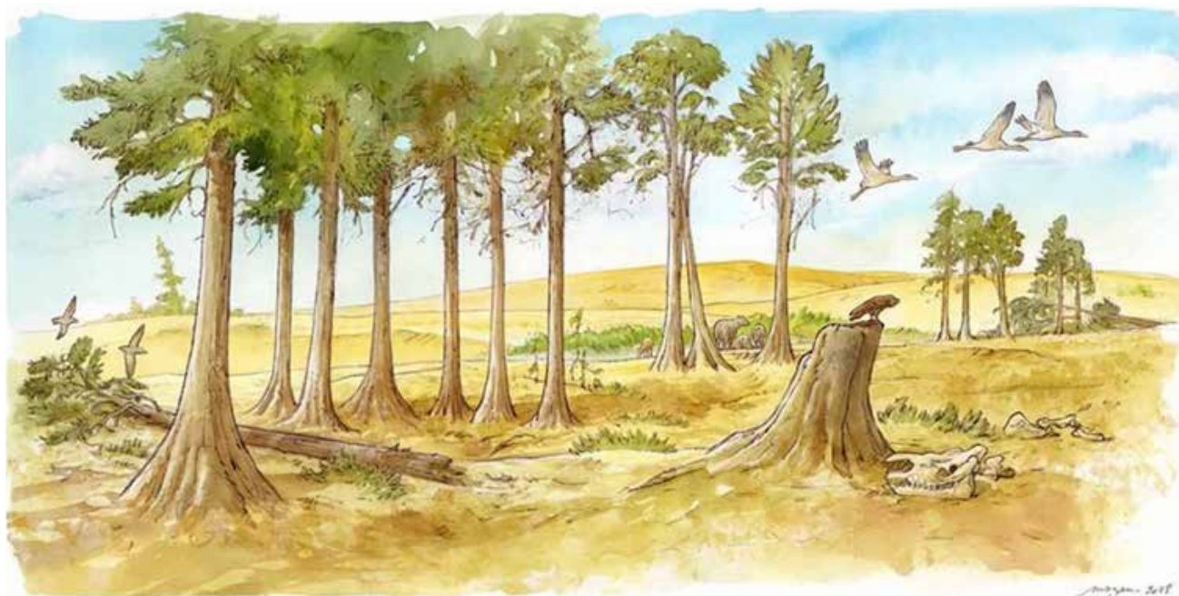
Reconstitution de l'écosystème de Villejust, il y a 30 millions d'années, à partir de l'étude des fossiles de la carrière du Bois de Lunézy.
